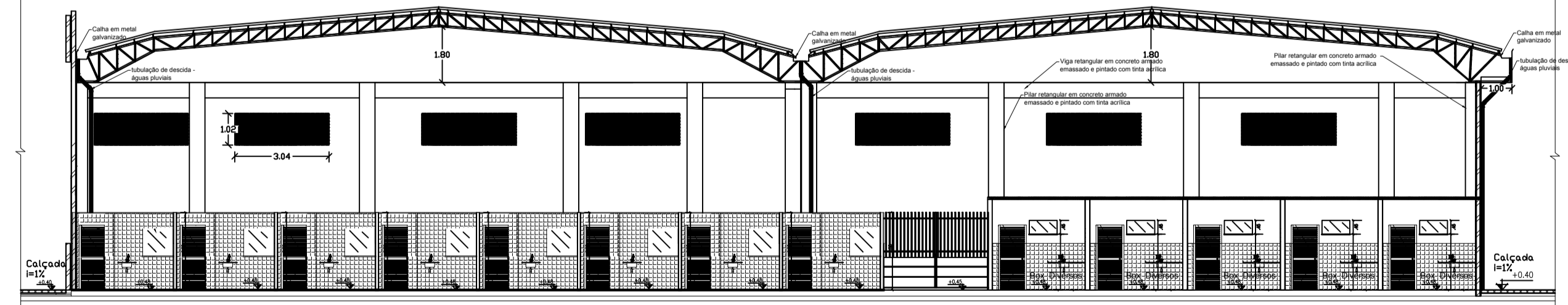
CORTE AA Escala: 1/100
